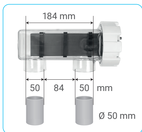
Elektroda TE-25
